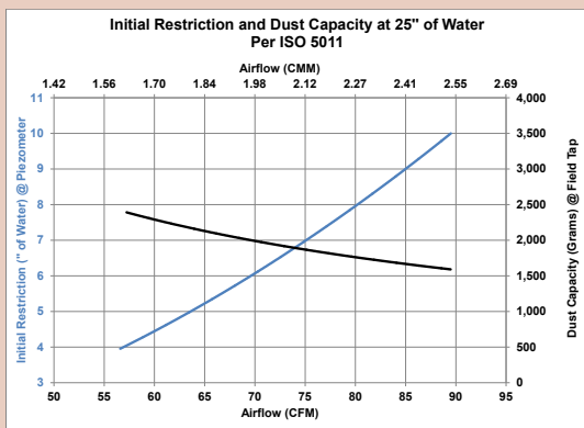
G052828 90° Outlet
